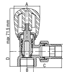
Вентиль ручной угловой Poker Plus
