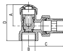
Вентиль обратный угловой Poker Plus
